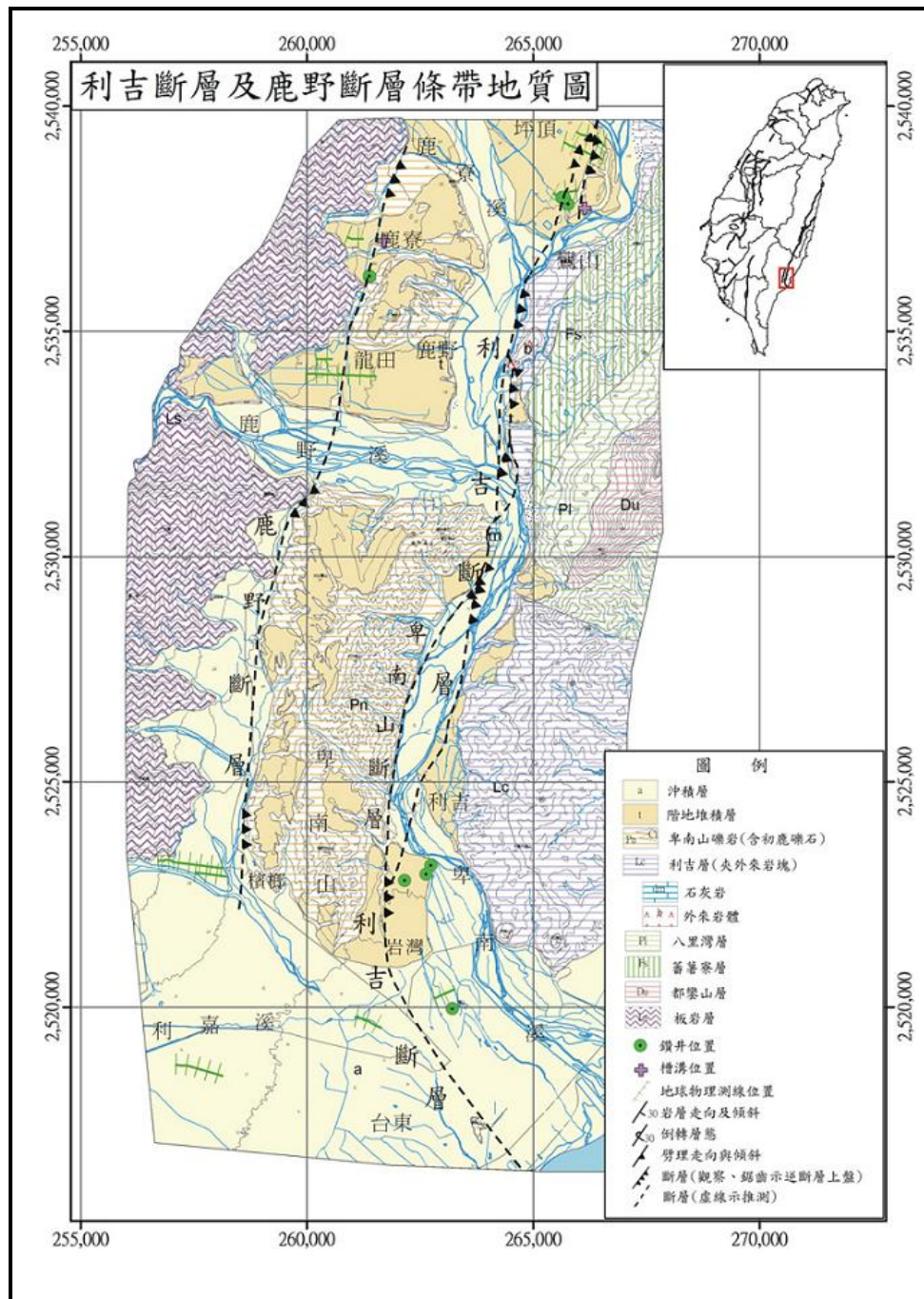
圖 1-6 利吉斷層及鹿野斷層條帶地質圖
